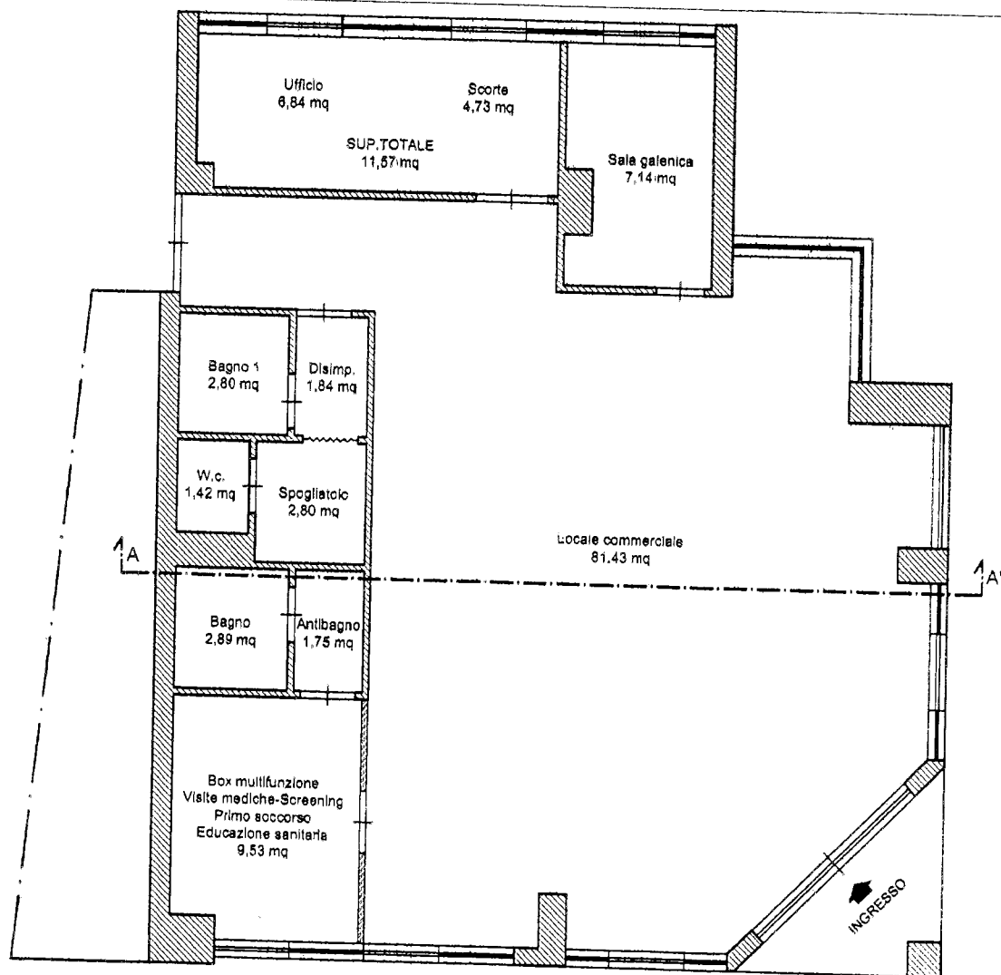
PIANTA SCALA 1:100
